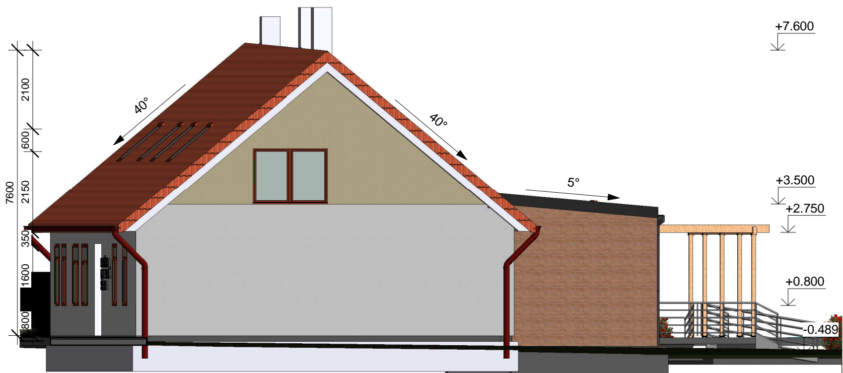
Juhozápadný pohľad
